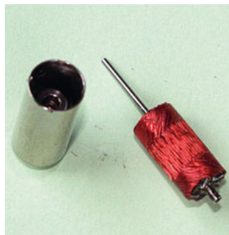
Servomotor mit herausgenommenem Glockenanker (Corless).
