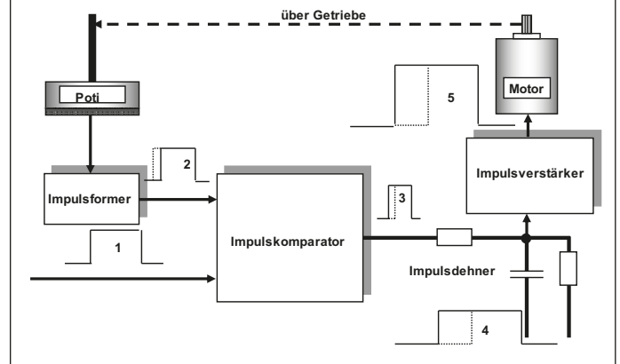
Impulsverlauf im Servoverstärker.
