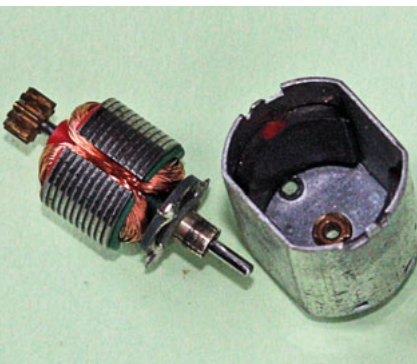
Zerlegter Servomotor mit Eisenanker.
