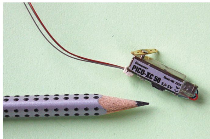
Frühe Miniaturisierungsversuche bei Servos.
