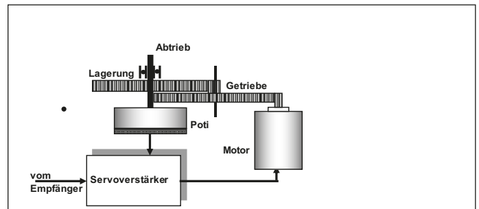
Prinzip eines analog arbeitenden Servos.
